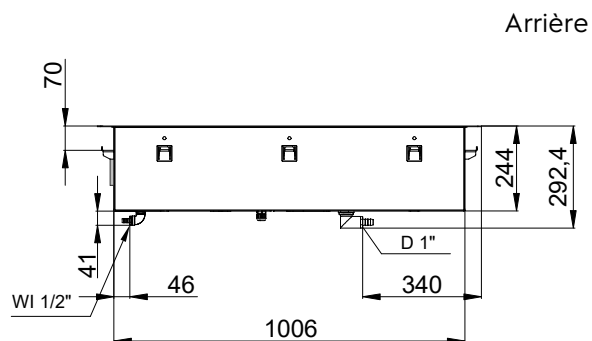
Côté
