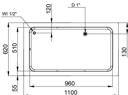
Dessus
